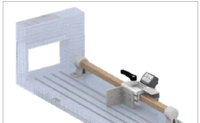
Messanschlag mit magnetischer Wegmessung
