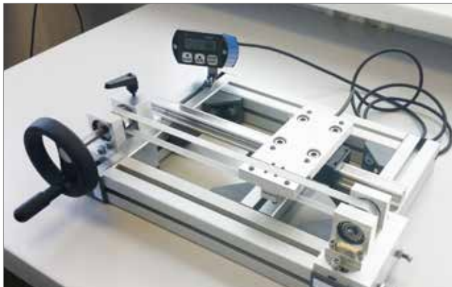
Positioniertisch Magnetisches Messsystem, batteriebetrieben
