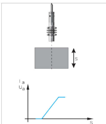
Annäherung in axialer Richtung
