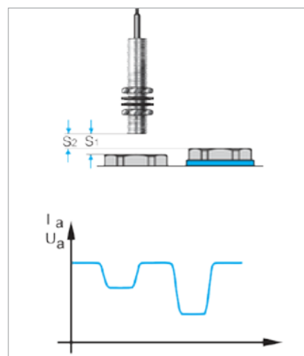
Erkennen von montierten Dichtringen
