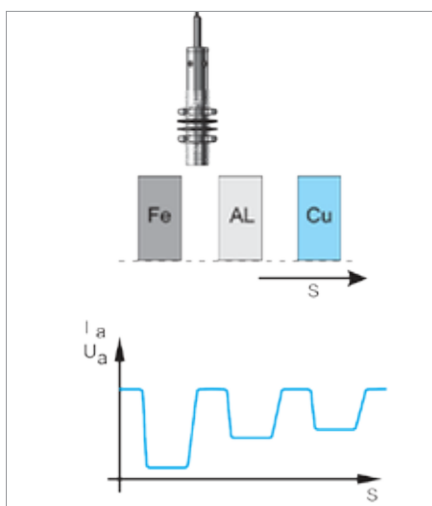
Erkennen unterschiedlicher Werkstoffe
