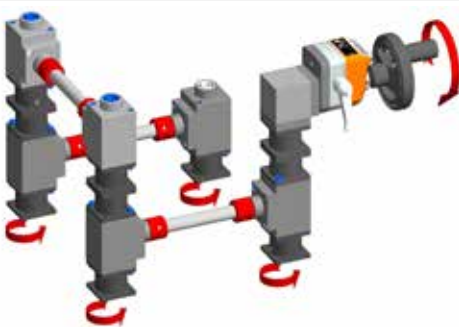
Winkelgetriebe 66/5
