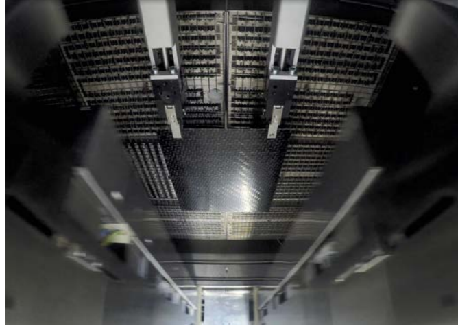
Kleiner CT LT-Messkopf mit Laminar-Freiblaseinrichtung in einer Thermoform-Maschine
