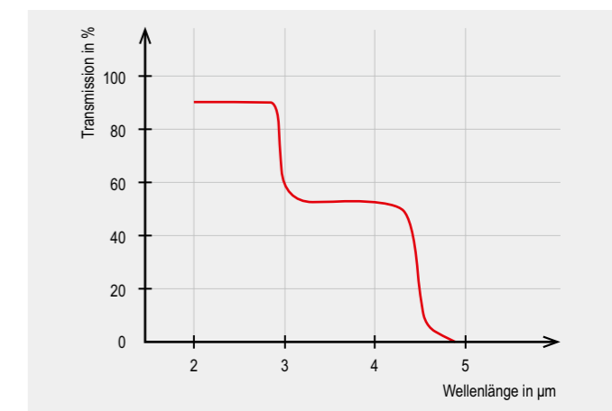
Spektrale Durchlässigkeit von Glas
