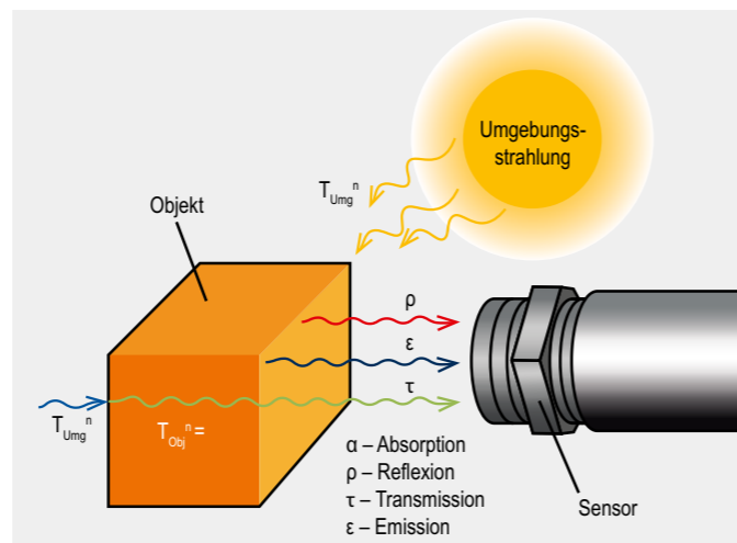
Umgebungsstrahlungskompensation
