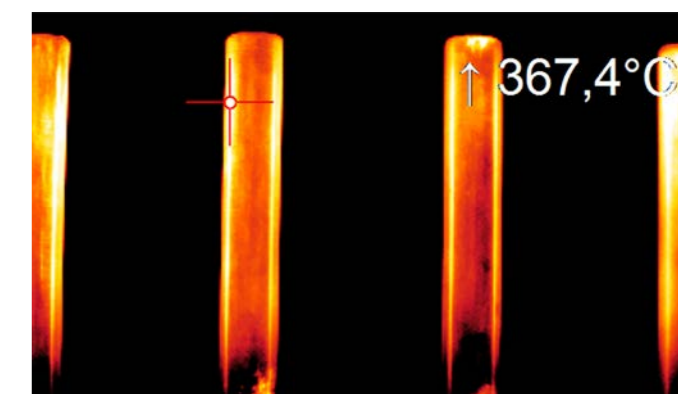
Hot-Spot-Messung an Glasröhren
